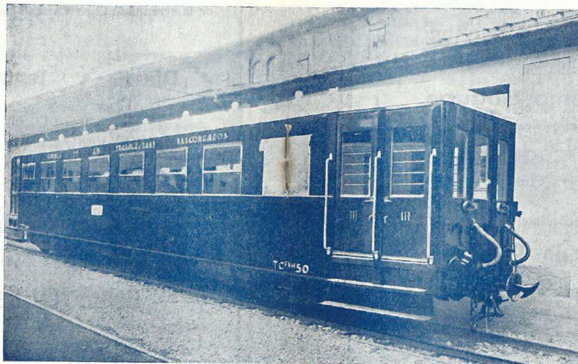
Coche de estructura metálica de III clase para viajeros, destinado a la Compañía de los Ferrocarriles Vascongados.
