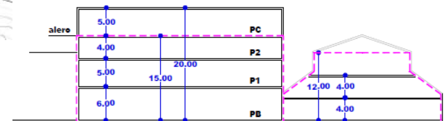
SEKZIO OROKORRA AA' SECCION TIPO AA'
