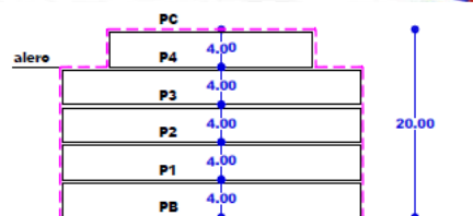
SEKZIO OROKORRA BB' SECCION TIPO BB'
