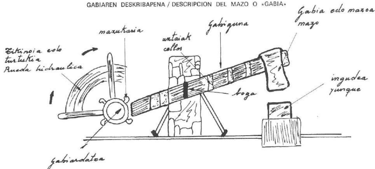
GABIAREN DESKRIBAPENA / DESCRIPCION DEL MAZO O «GABIA»
