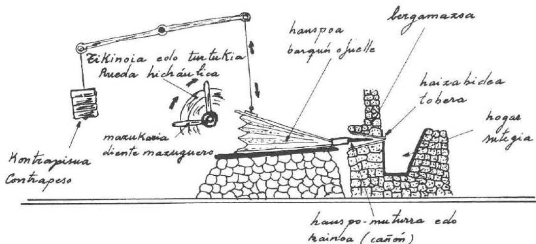
GABIAREN DESKRIBAPENA / DESCRIPCION DEL MAZO O «GABIA»
