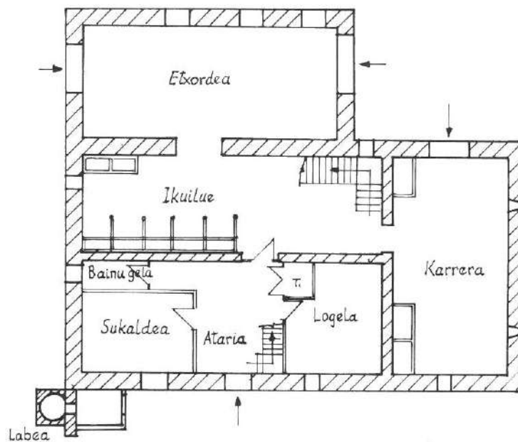
PLANTA BAJA - BEHE OINA
