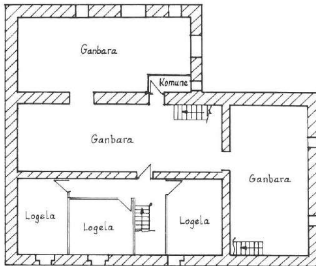
PLANTA PRIMERA - LEHEN OINA
